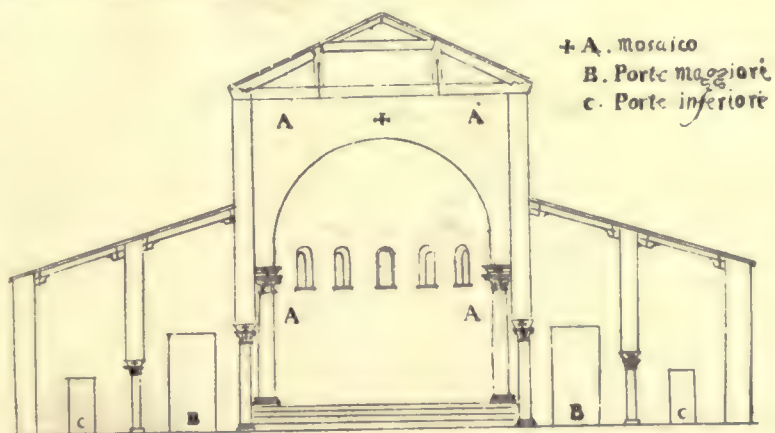
Fig. 3.—Ravenna. Basilica Ursiana. Section (370-384). (From Buonamici, "Metropolitana di Ravenna.")
